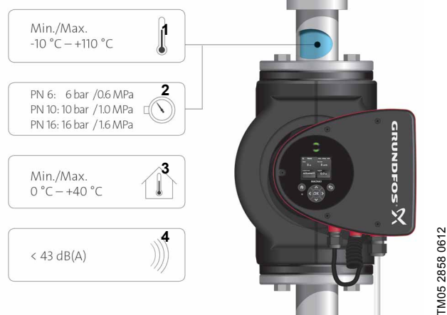
Рис. 3 Условия эксплуатации
